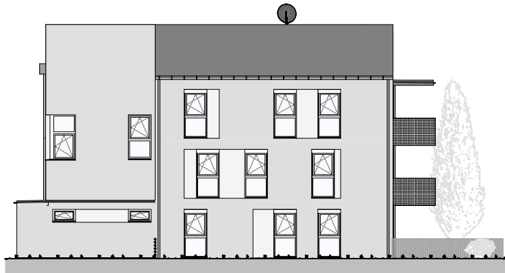
ANSICHT NORD
