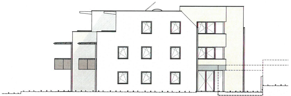
ANSICHT OST
