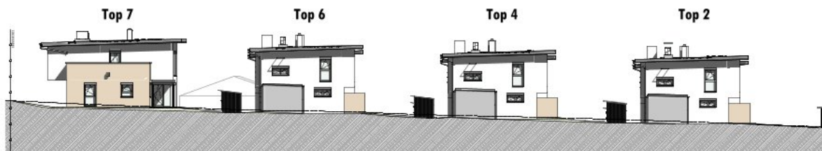
Südwestansicht
