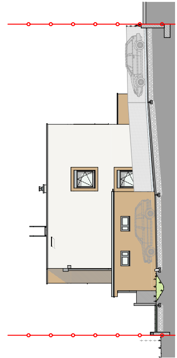
ANSICHT NORD
